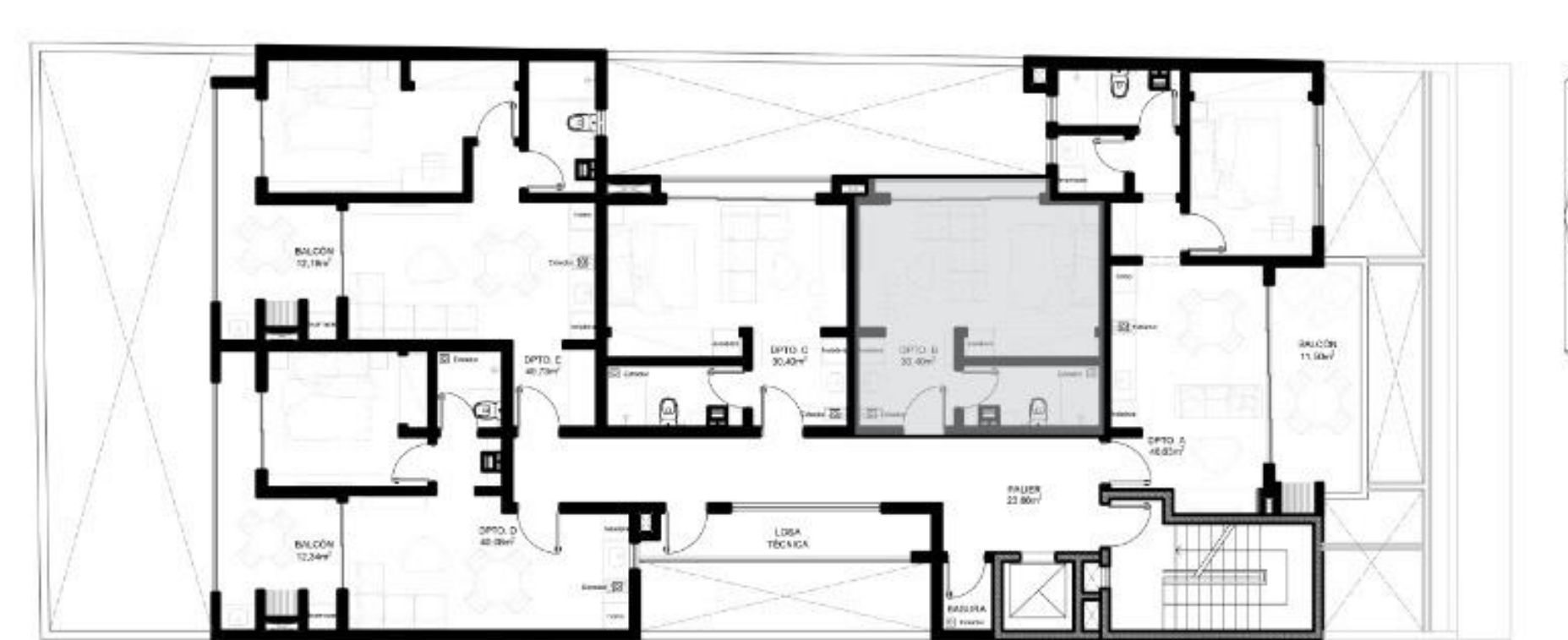
PLANTA TIPO 1m 5m 10m
